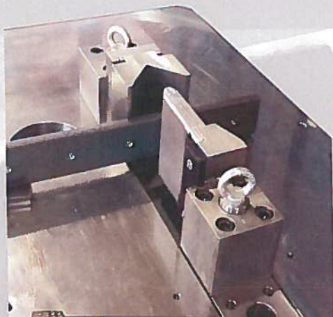
Vue du poste de commande et des coupleurs hydrauliques
